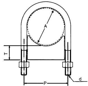
"UP" タイプ
