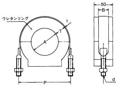
"MS" タイプ
