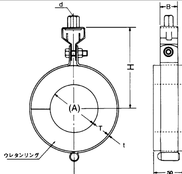
"AG" タイプ
